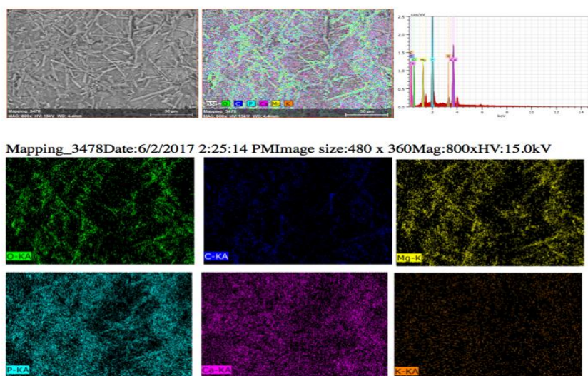
รูปที่ 4-18 ผลการวิเคราะห์ธาตุโดยใช้เทคนิค EDX ของตัวอย่างน้ำหลังกระบวนการที่มีค่า pH = 9.00
