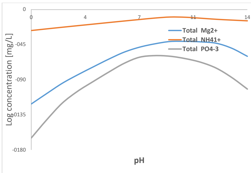
รูปที่ 4.7 ผลการจำลองหาสถานะที่เหมาะสมสำหรับการตกตะกอนปุ๋ยสูตรไวท์โดยใช้โปรแกรมสมดุลทางเคมี MINTEQ
